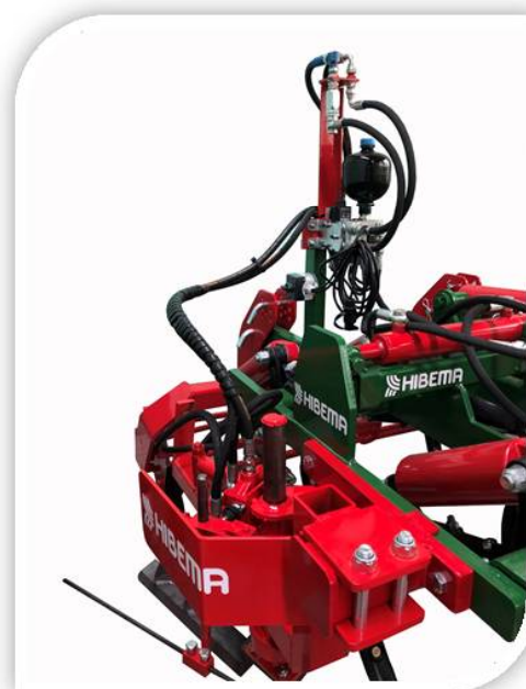
Intercepa mixto con palpador, válvula Bypass y mando electro-hidraulico
