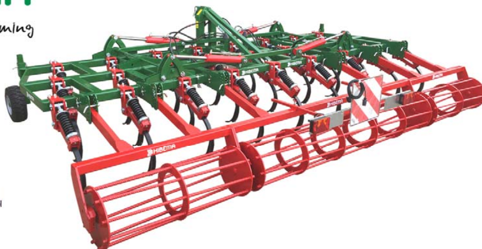
CM-25 SH (3F) Rodillo+ Kit de luces Pleg. 4 cilindros, ruedas de control
